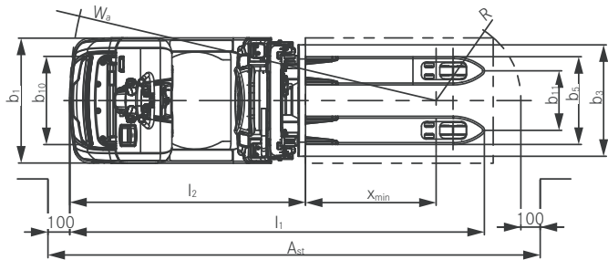
Draufsicht OPX-D 20
