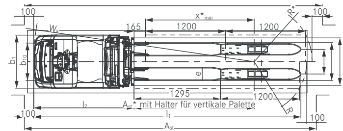
Draufsicht OPX-L 20
