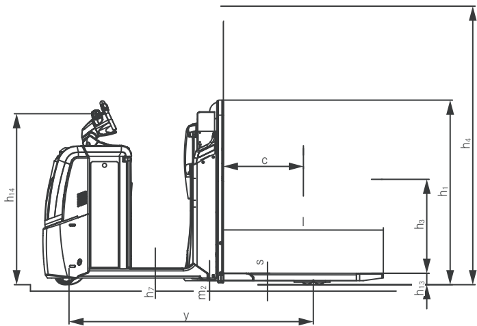
Seitenansicht OPX-L 12
