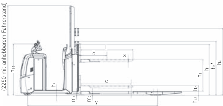
Seitenansicht OPX-L 20
