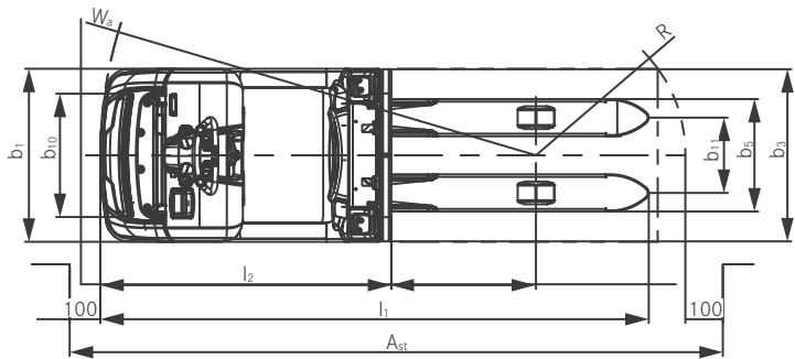
Draufsicht OPX-L 12
