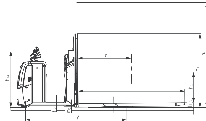
Seitenansicht OPX-L 16
