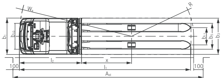
Draufsicht OPX-L 16
