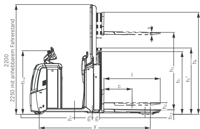
Seitenansicht OPX-D 20
